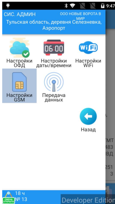
Меню Настройки ККТ
